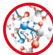
AMINOÁCIDOS LEVÓGIROS
